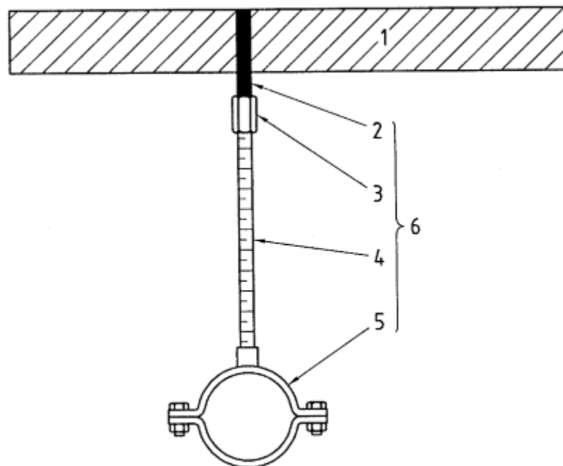
Hình 1 - Một số kiểu thiết bị giá treo ống
