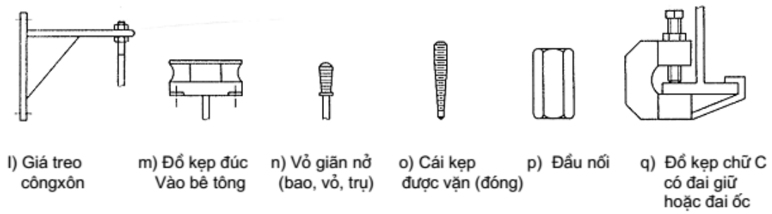
Hình 1 - Một số kiểu thiết bị giá treo ống
